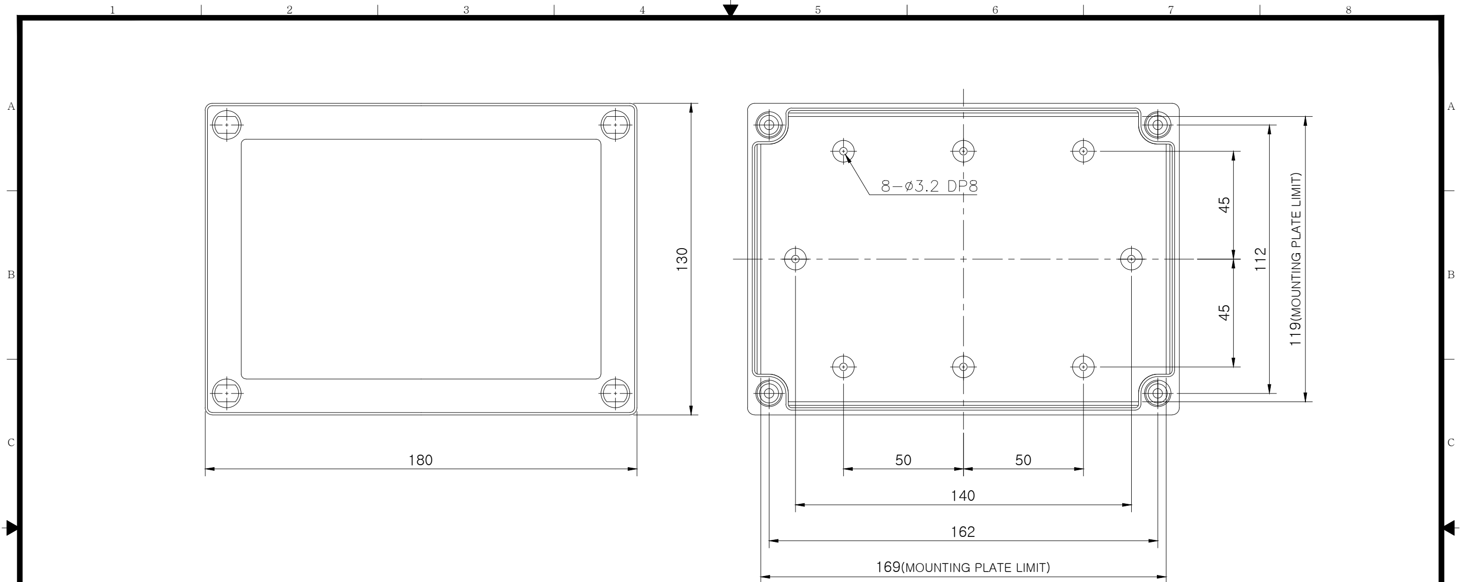
SECTION A-A
